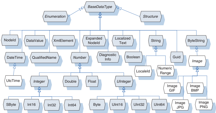
Fig. C.2 DataType Hierarchy
