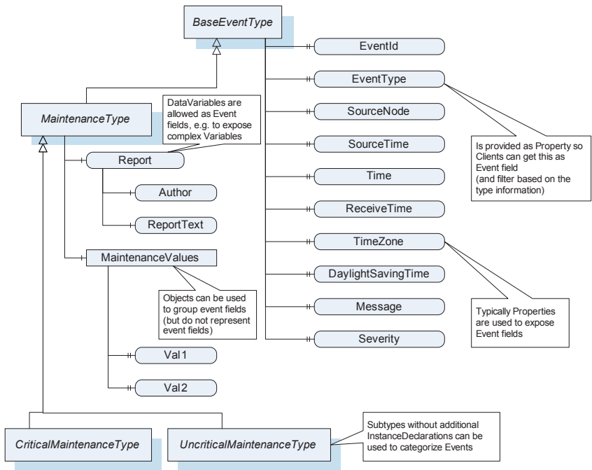
Fig. 2.44 EventType hierarchy
